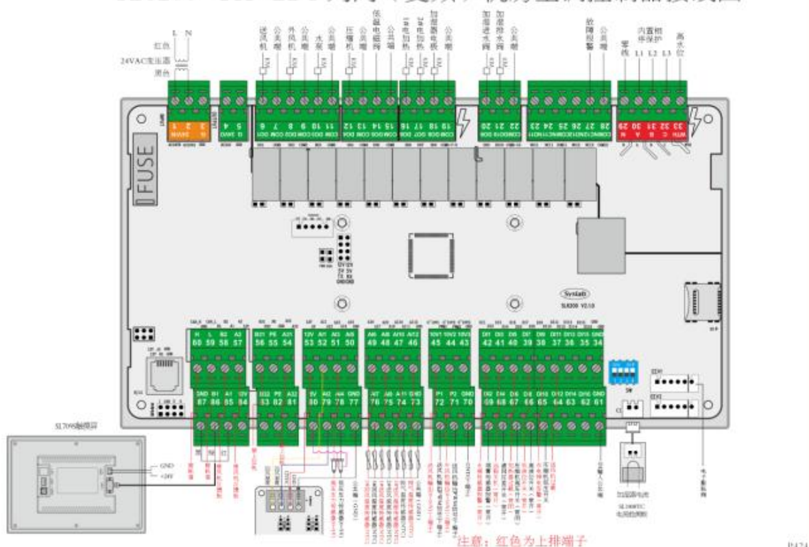
SL6200-TH-LDS 列间（变频）机房空调控制器接线图
