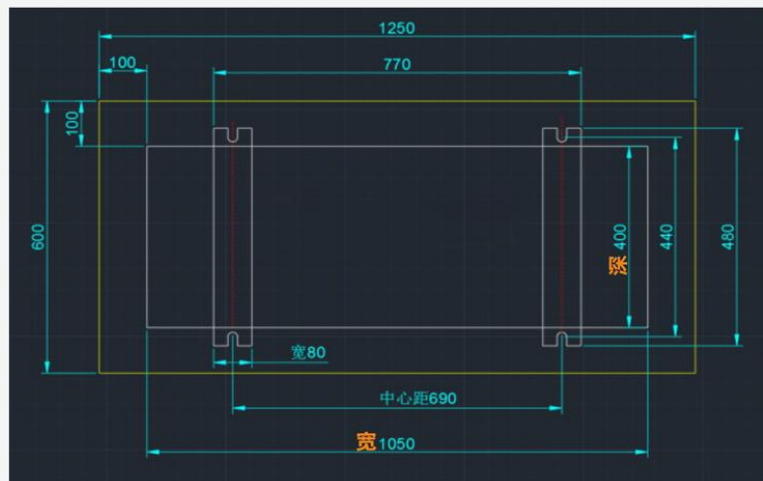
选配 立式外机 底座规格
